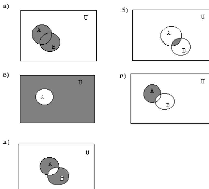
Рис. 1. Графическое изображение алгебраических операций над множествами A и B .
