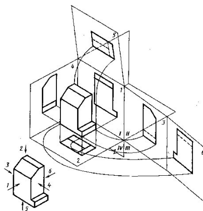
Рис.8. Прямоугольное проецирование
