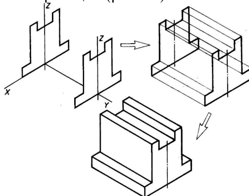
Рис. 12. Построение изометрической проекции
