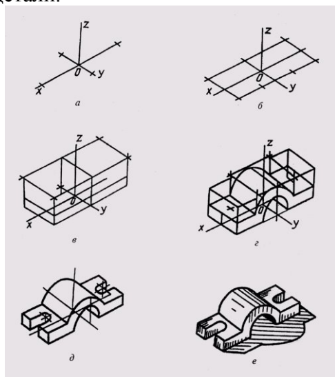
Рис.11.Изометрические проекции
