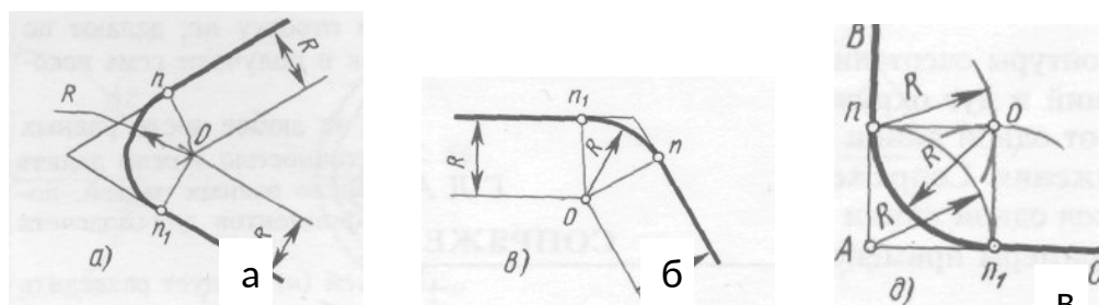
Рис.5. Сопряжения углов а – острого; б – тупого; в – прямого.
