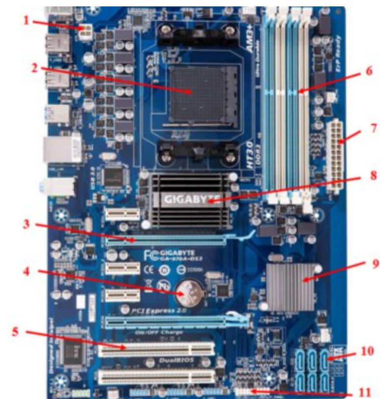
Рисунок 1 – Материнская плата
