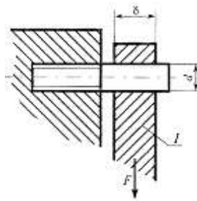
Рис.3. Шпилечное соединение.
