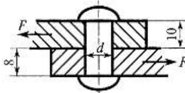
Рис.2.Заклёпочное соединение.
