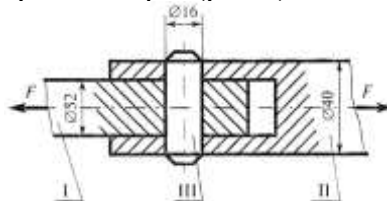
Рис.7. Штифтовое соединение.
