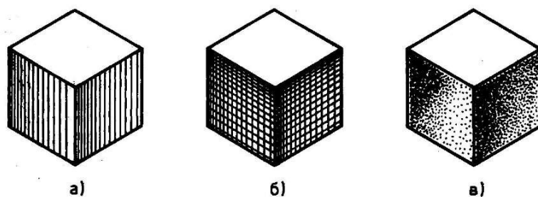
Рис. 9. Технические рисунки с выявлением объема шатировкой (а), шраффировкой (б) и точечным оттенением (в)
