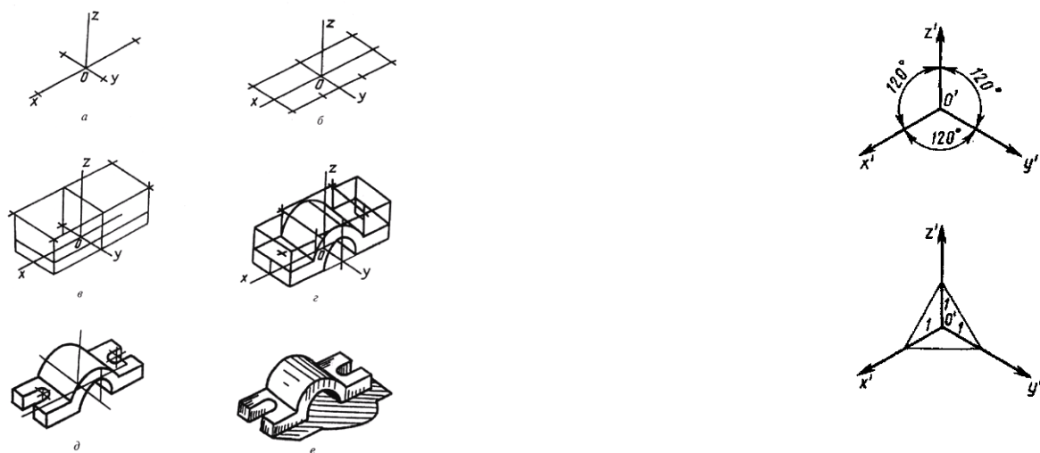
Рис.11.Изометрические проекции
