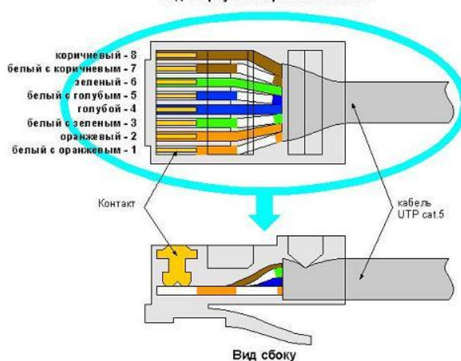
Рис.7. Порядок разводки проводов витой пары по стандарту EIA/TIA568B.
