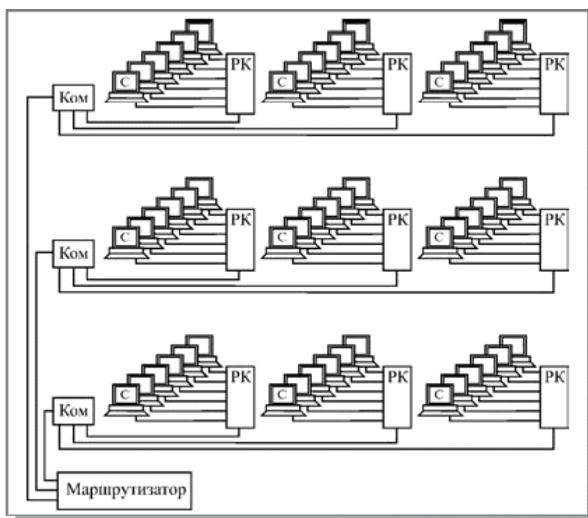
Рис. 2. Структура сети предприятия (С – серверы рабочих групп, ПК – репитерные концентраторы, Ком – коммутаторы)
