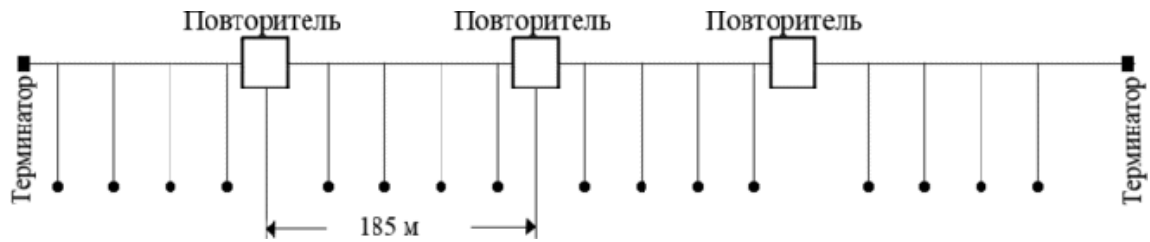
Рис. 4. Соединение сегментов в шинной топологии
