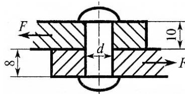
Рис.2.Заклёпочное соединение.
