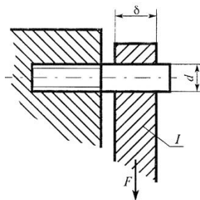
Рис.3. Шпилечное соединение.
